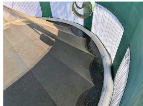
Figur 42: Aquatraz 4 med heist not.
