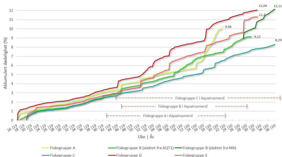
Figur 45: Akkumulert dødelighet for alle merder hvor det andre biologiprogrammet og tetthetsprogrammet ble gjennomført. Aquatrazmerder i grøntonner, konvensjonelle i rødtonner. Fiskegruppe A, B og C sto i Aquatrazmerd i deler av produksjonstida, indikert på figuren. Fiskegruppe C var gjenstand for fullstendig biologiprogram hvor fiskegruppe E var kontrollmerd.
