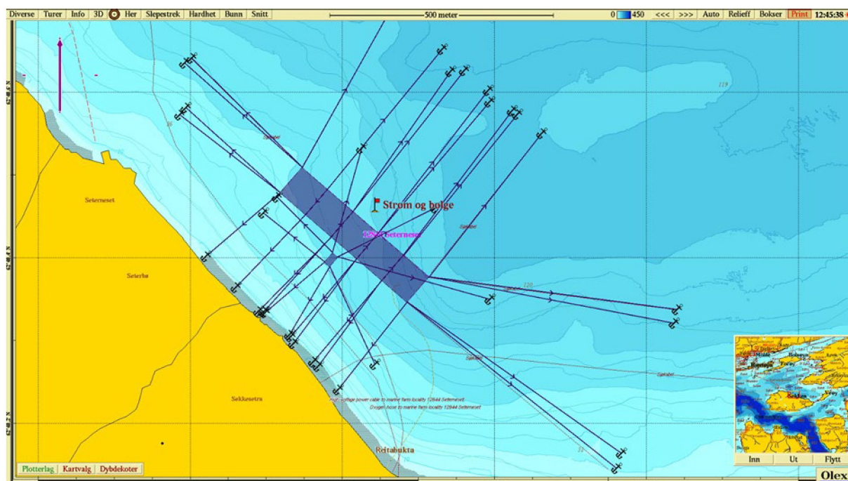
Figur 15 Plassering av strøm og bølgemåler på lokalitet Seterneset.
