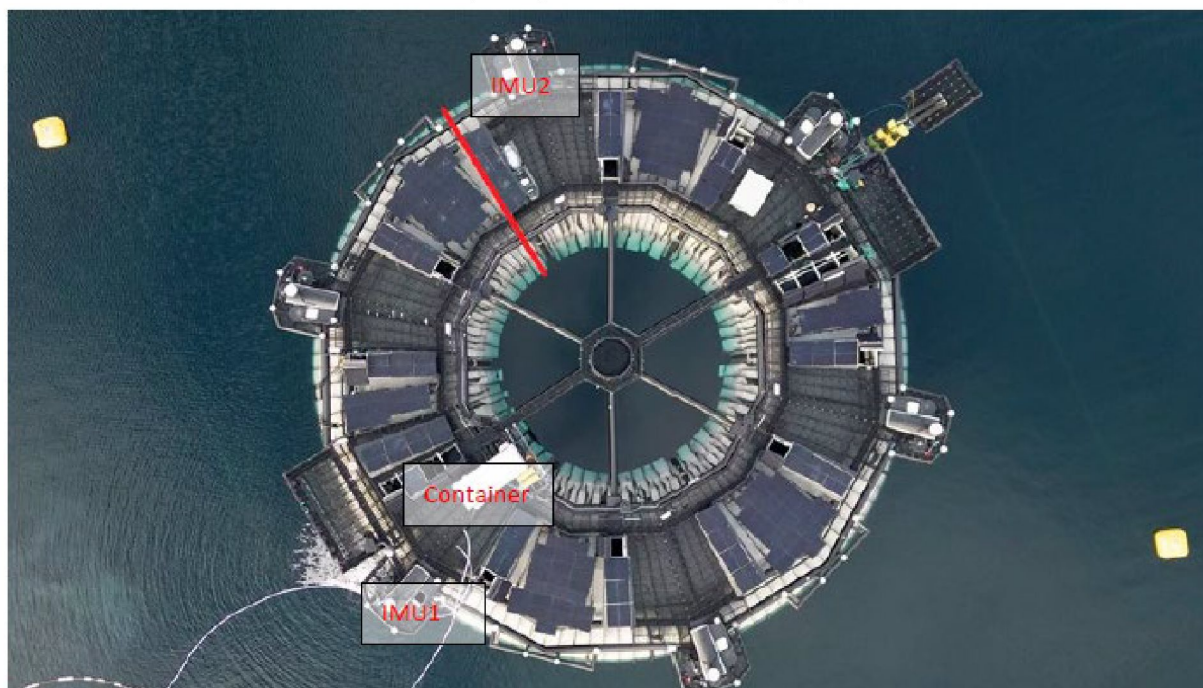
Figur 17 Flyfoto av Marine Donut med plassering av GPS og IMU'er
