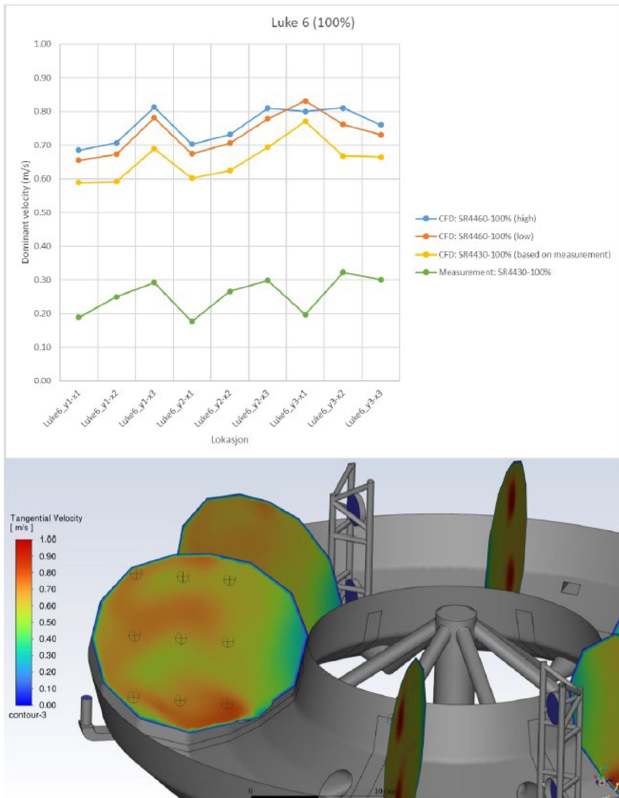
Figur 13 Luke 6 (100%) - dominerende hastighet; CFD vs. måling/2/
