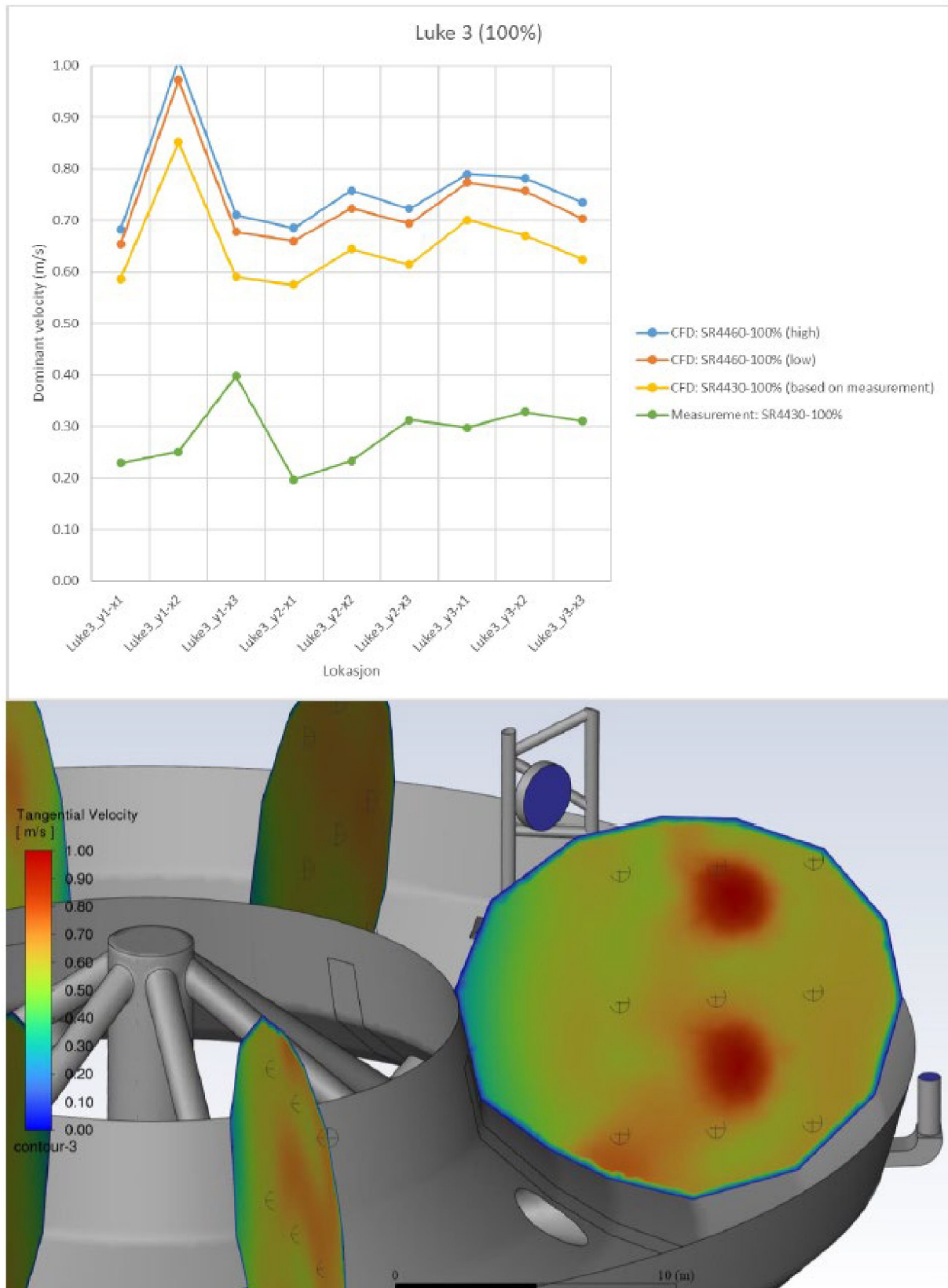
Figur 12 Luke 3 (100%) - dominerende hastighet; CFD vs. måling /2/
