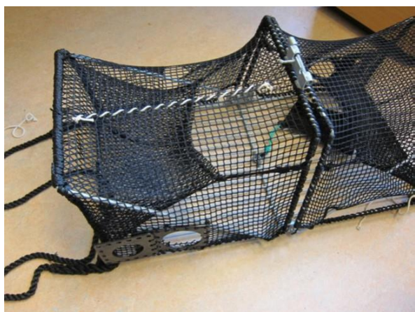
Figur 1. Rømmingshullet skal lages i taket eller i en sideflate på teinen. Snittet lisses sammen med bomullstråd. Bomullstråden skal kun knytes i endene.
