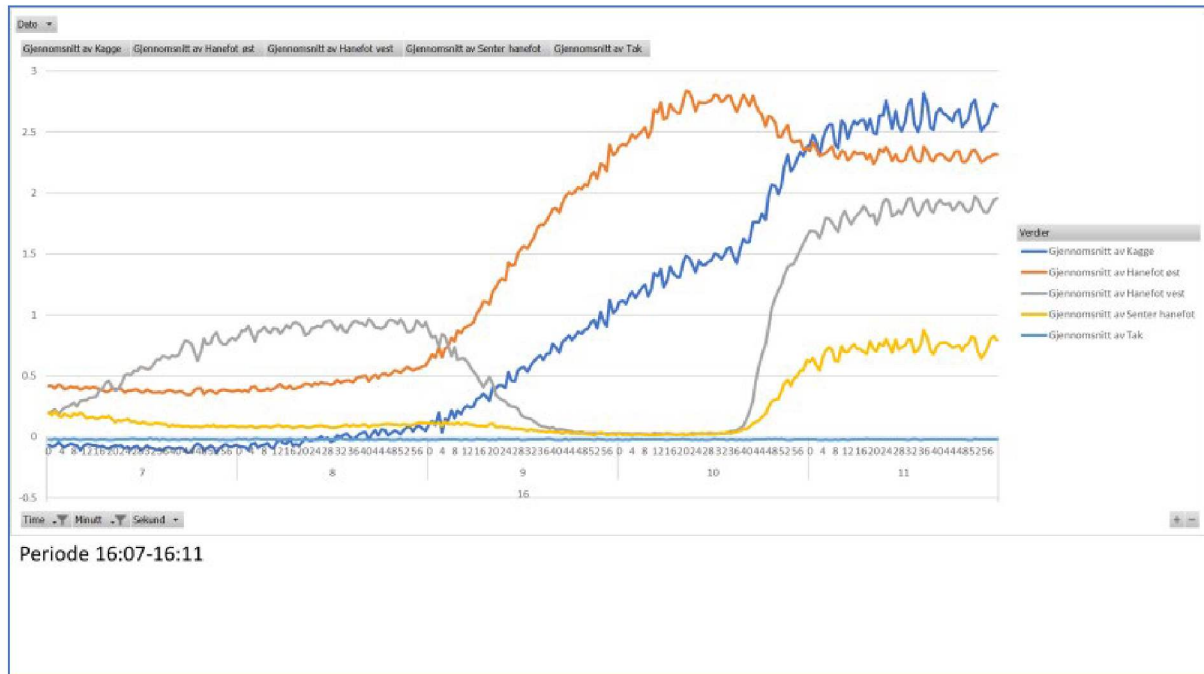
Figur 11 Krefter i lastsjakler under senking av merden
