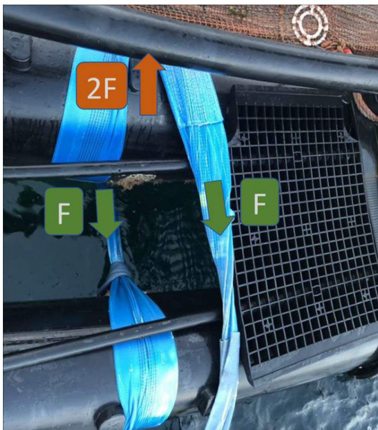
Figur 18 Kraftbilde på indre flyterør
