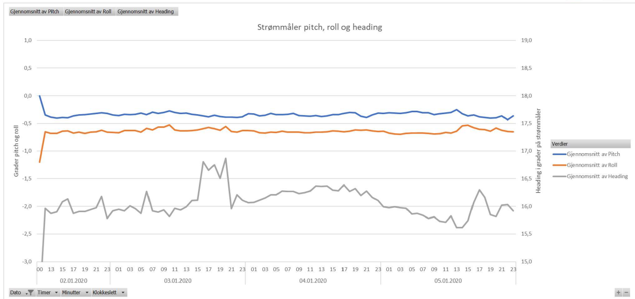
Figur 8 Måling av pitch, roll og heading i strømmåler montert på luftkuppel.
