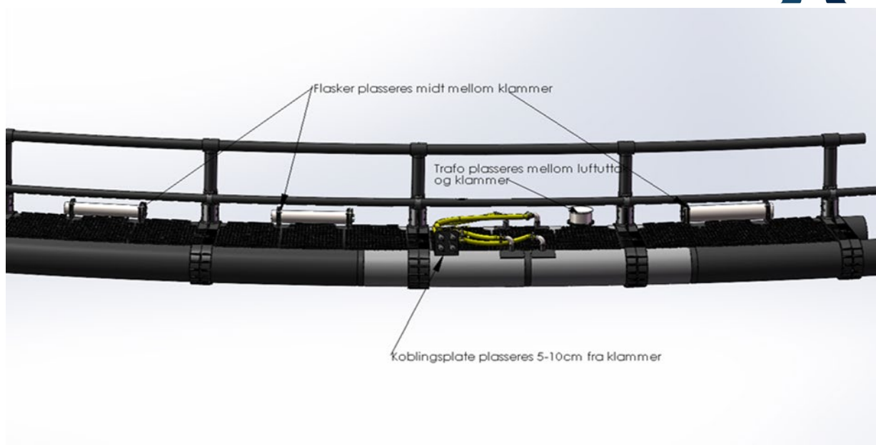
Figur 3 Luftsider med kontrollsyndere og trafo
