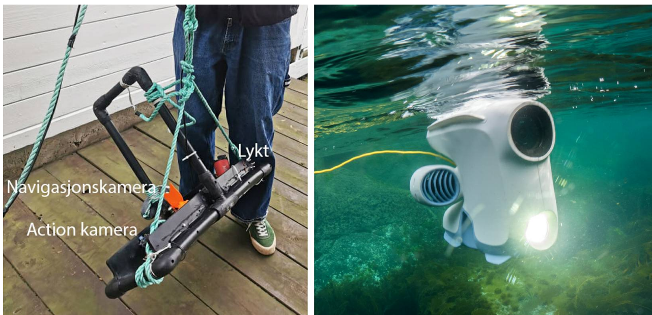
Figur 7. Venstre: Eksempel på videorigg med undervannsløkt, kablet navigasjonskamera og fastmontert action kamera. Høyre: Eksempel på mindre undervannsdrone (Foto: Jonas Follesø).
